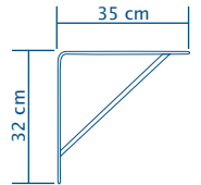
Mão Francesa TRIÂNGULO
