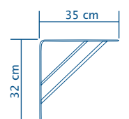
Mão Francesa TRIÂNGULO PARALELA
