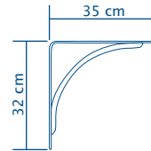
Mão Francesa ARCO
